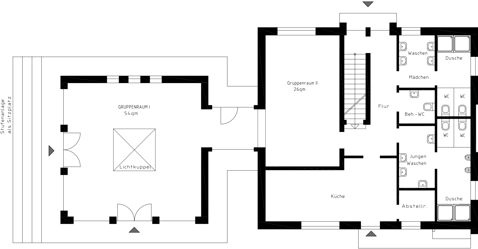
Grundriss Erdgeschoß
