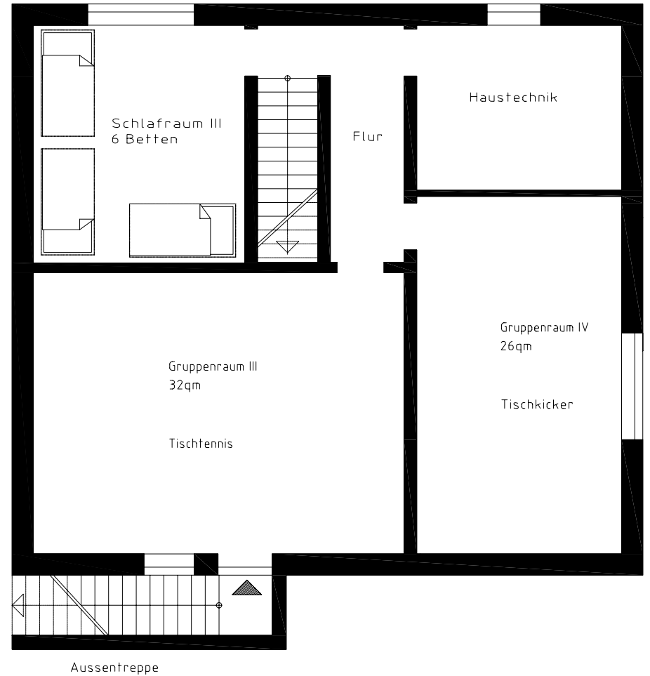
Grundriss Kellergeschoß
